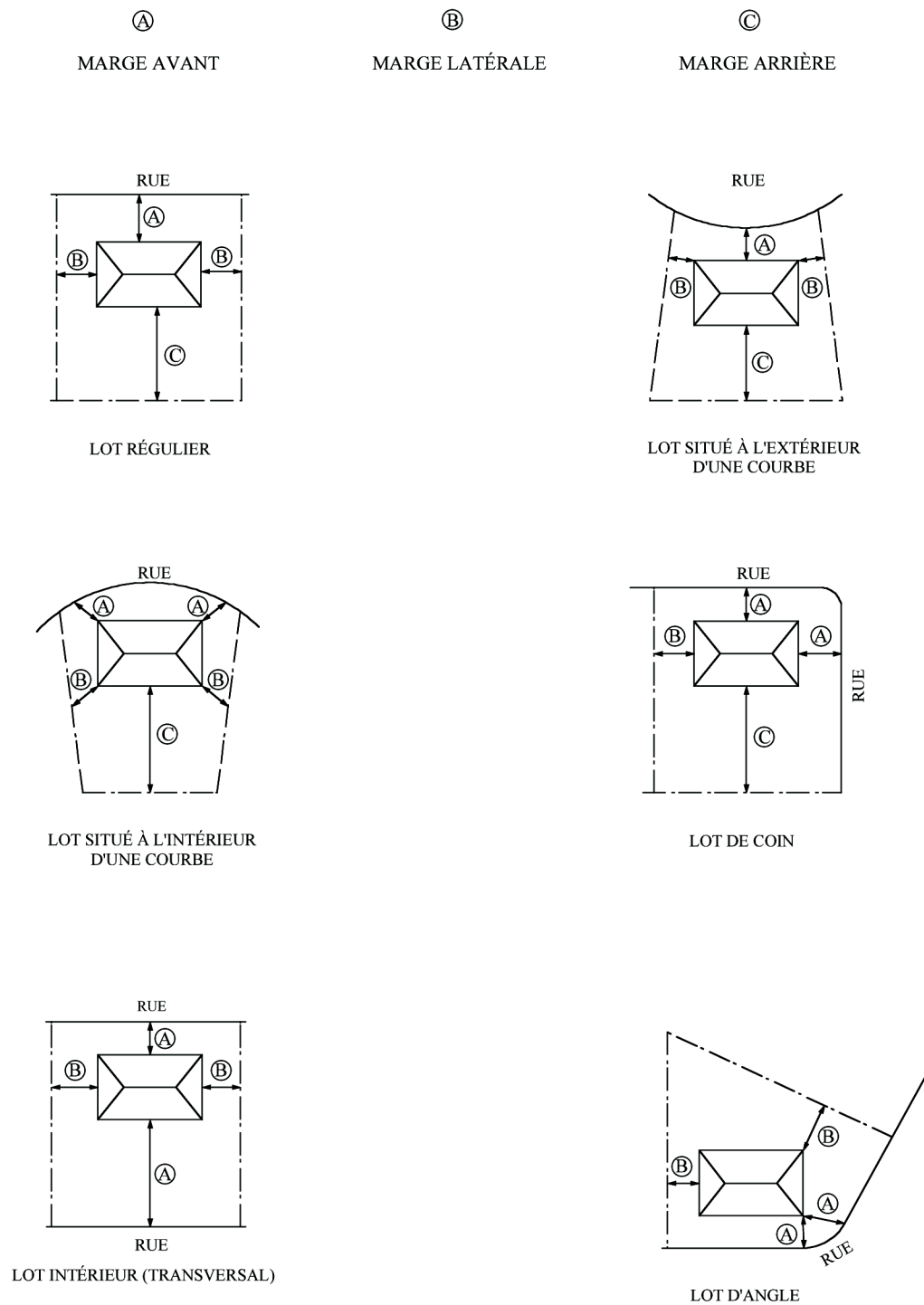
FIGURE 3 : MARGES DE RECUL AVANT, LATÉRALE ET ARRIÈRE
